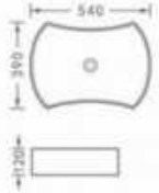
YJ-607
