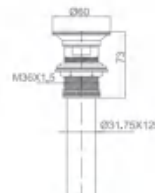
B016A-05 Flip plug waste 翻板去水
